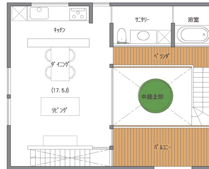
■2階平面図
